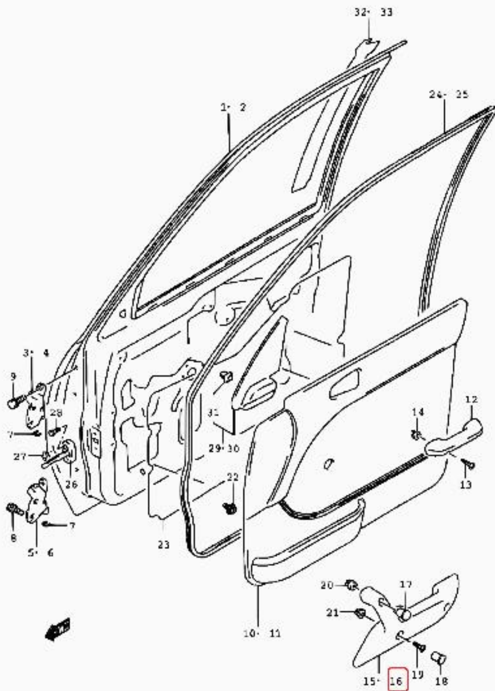
SP416-4 E66_214 5DR FRONT DOOR PANEL
