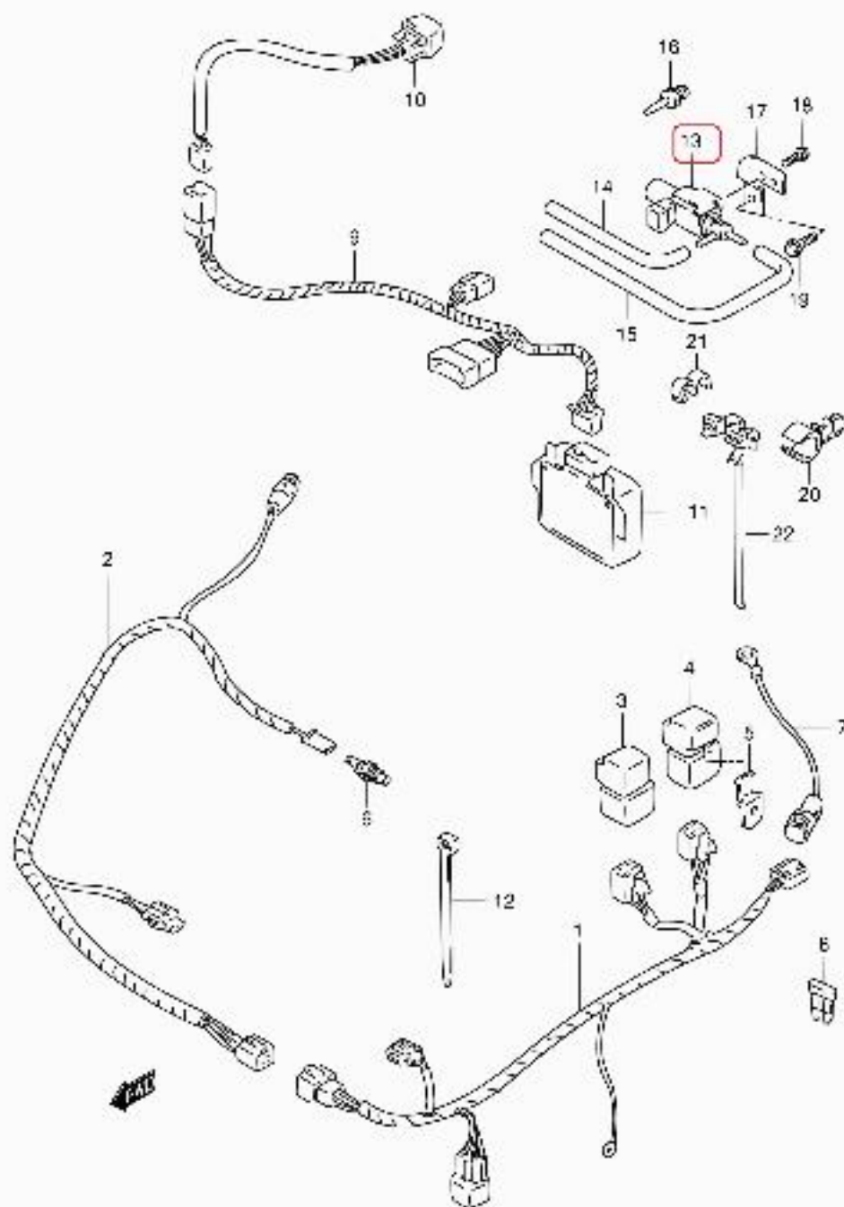
SE416 4 E01 249 A/C WIRING HARNESS(RHD)
