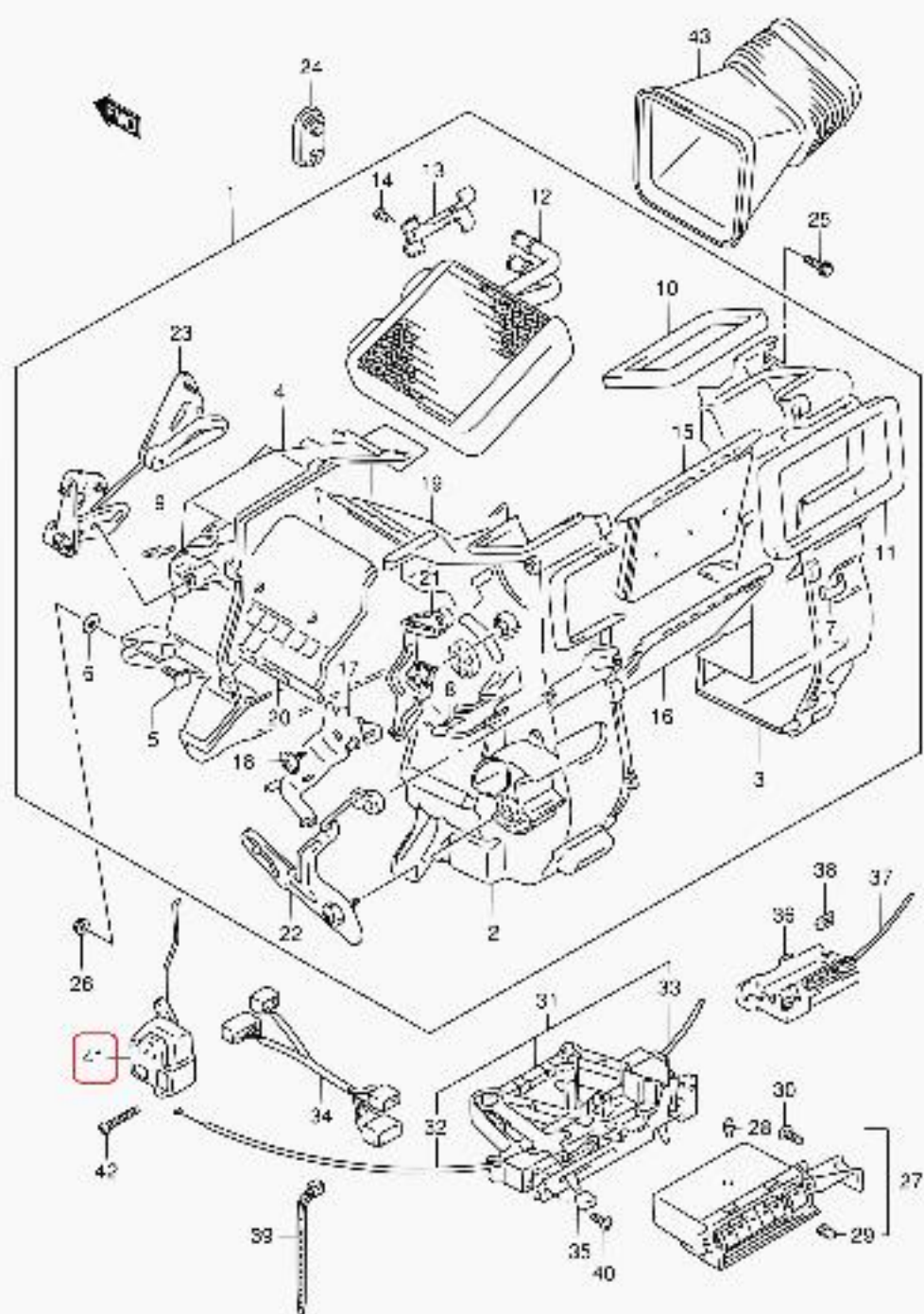
SE416 4 E01 194A HEATER (TYPE 5 LHD)
