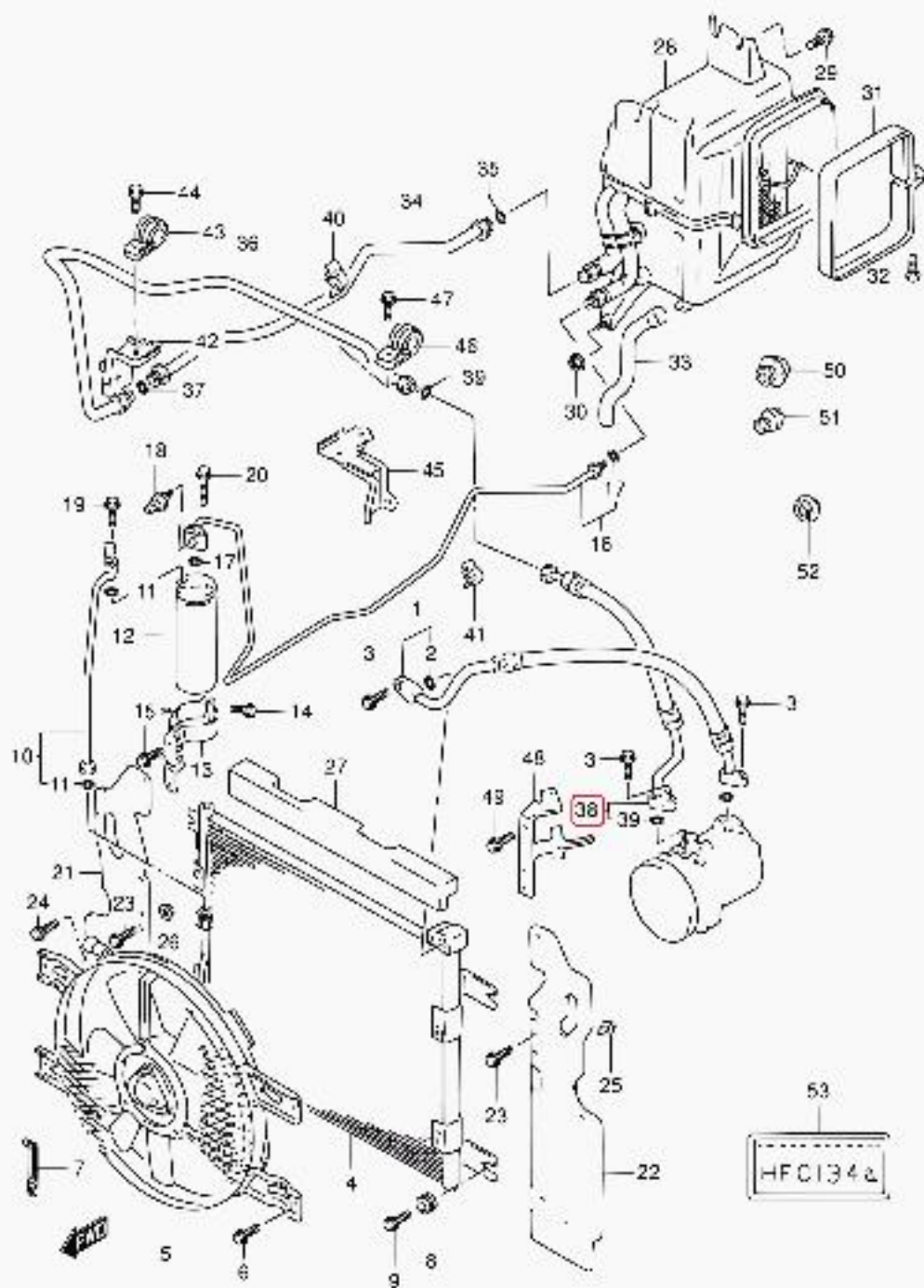
SV620 3 E01 246 AIR CON PIPING(LHD)
