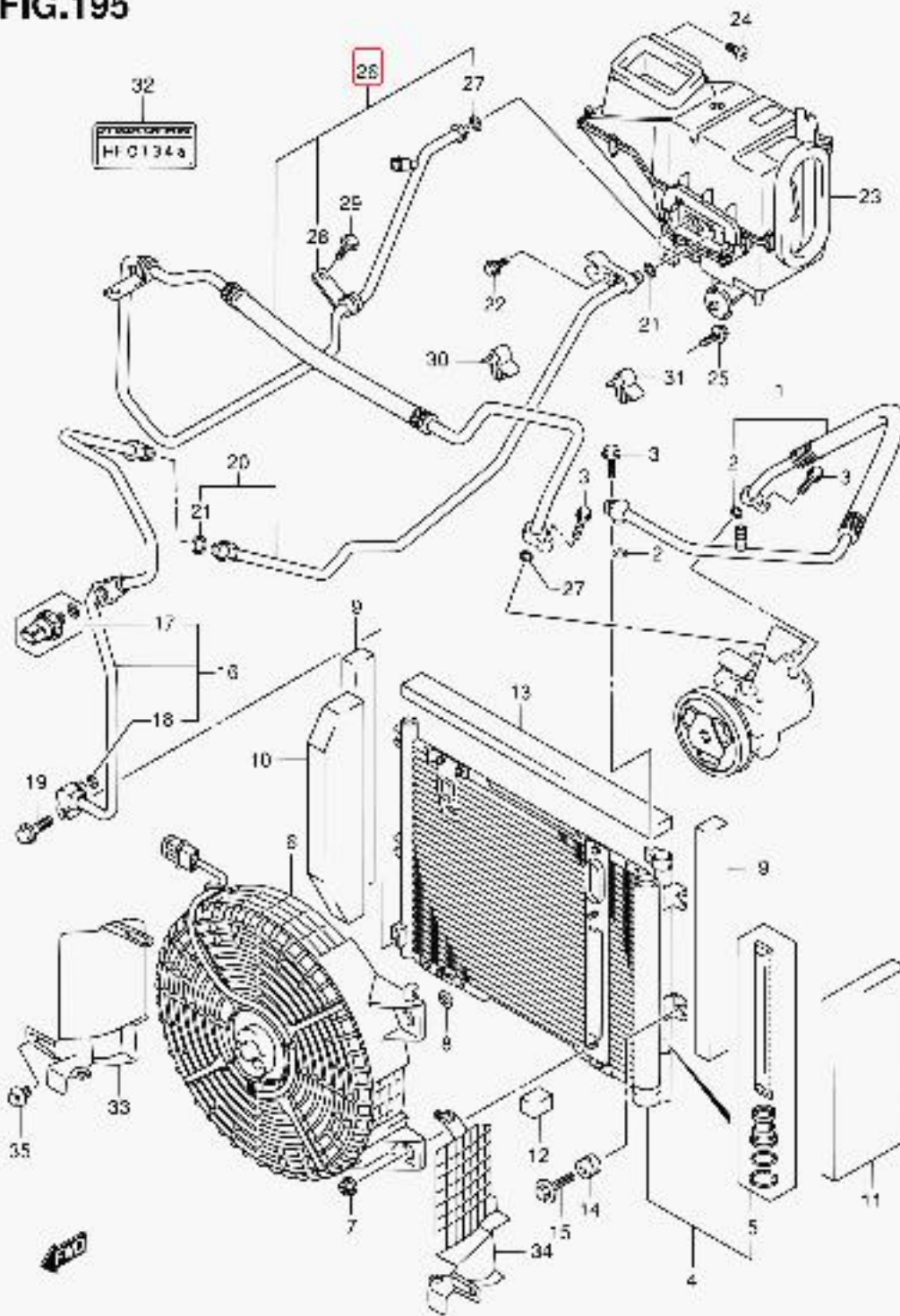
SN413V-5 E22 195 AIR CON PIPING (1)
