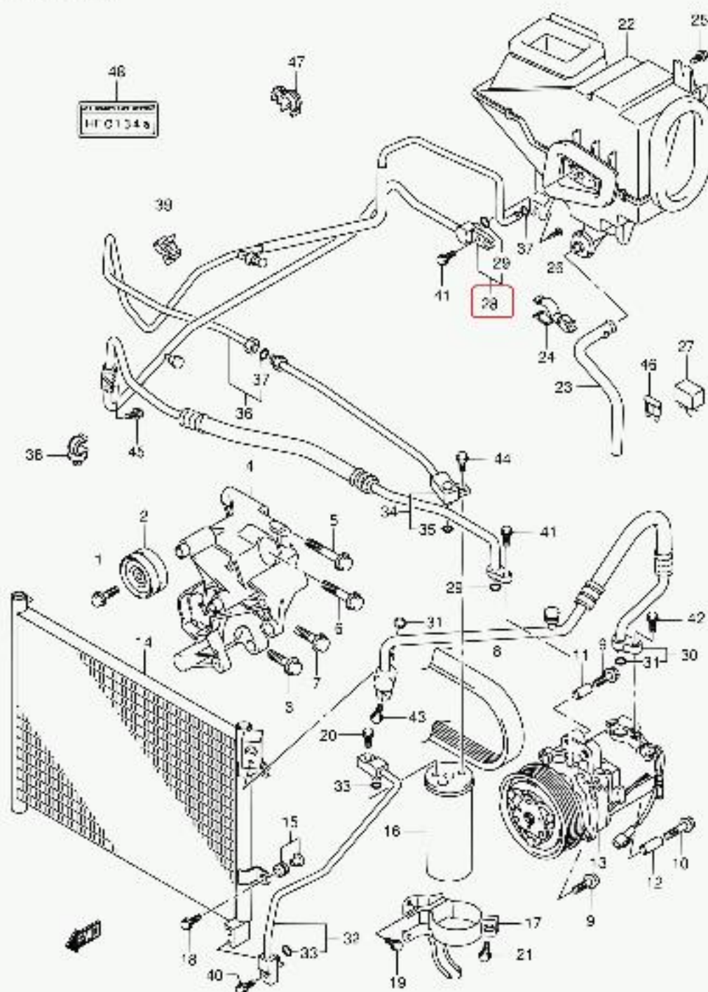
SA413V-5 E22 196 AIR CON PIPING (2)
