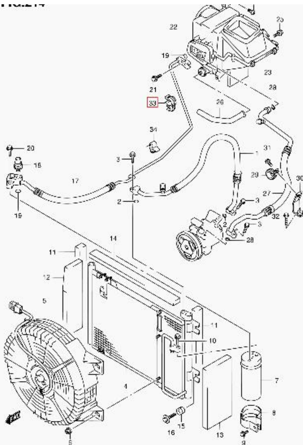
SA413V-2 E22 214 AIR CON PIPING (3)
