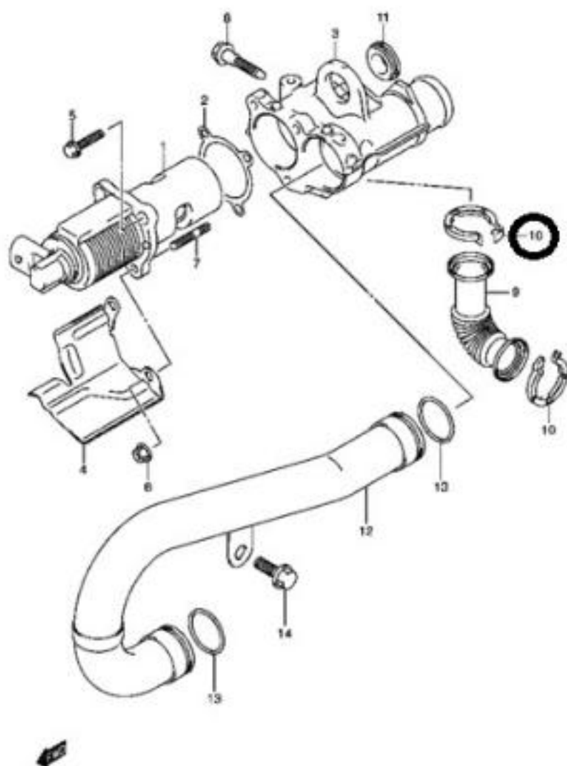
SN413V-5 E22_049 EGR VALVE (SN415VD:1)
