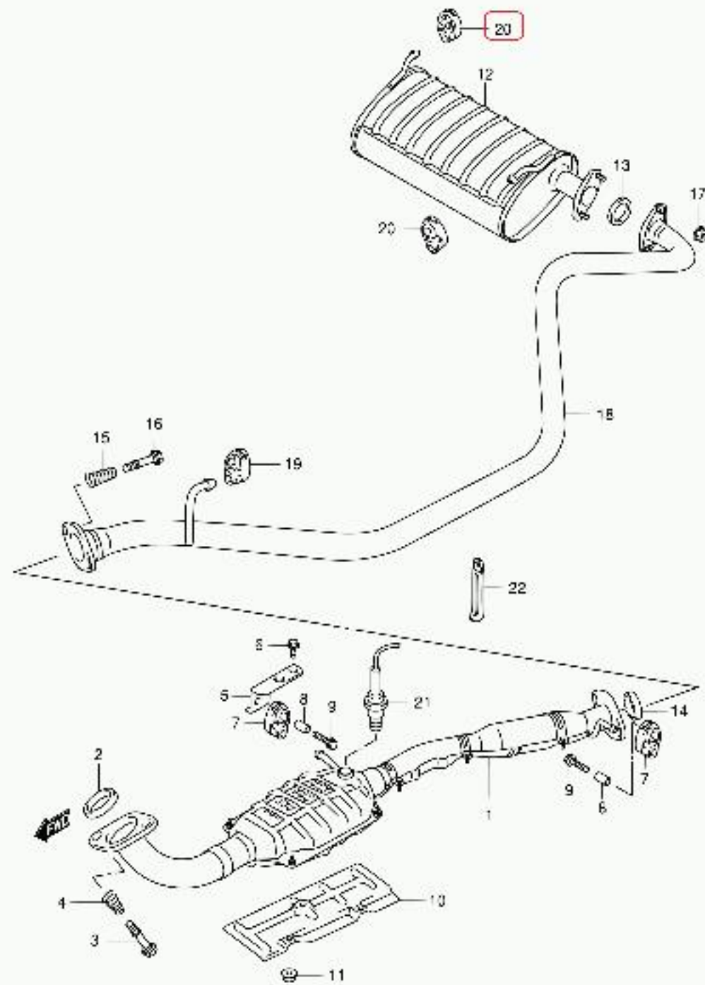
SN413V-2 E22 025 MUFFLER (SN413V)
