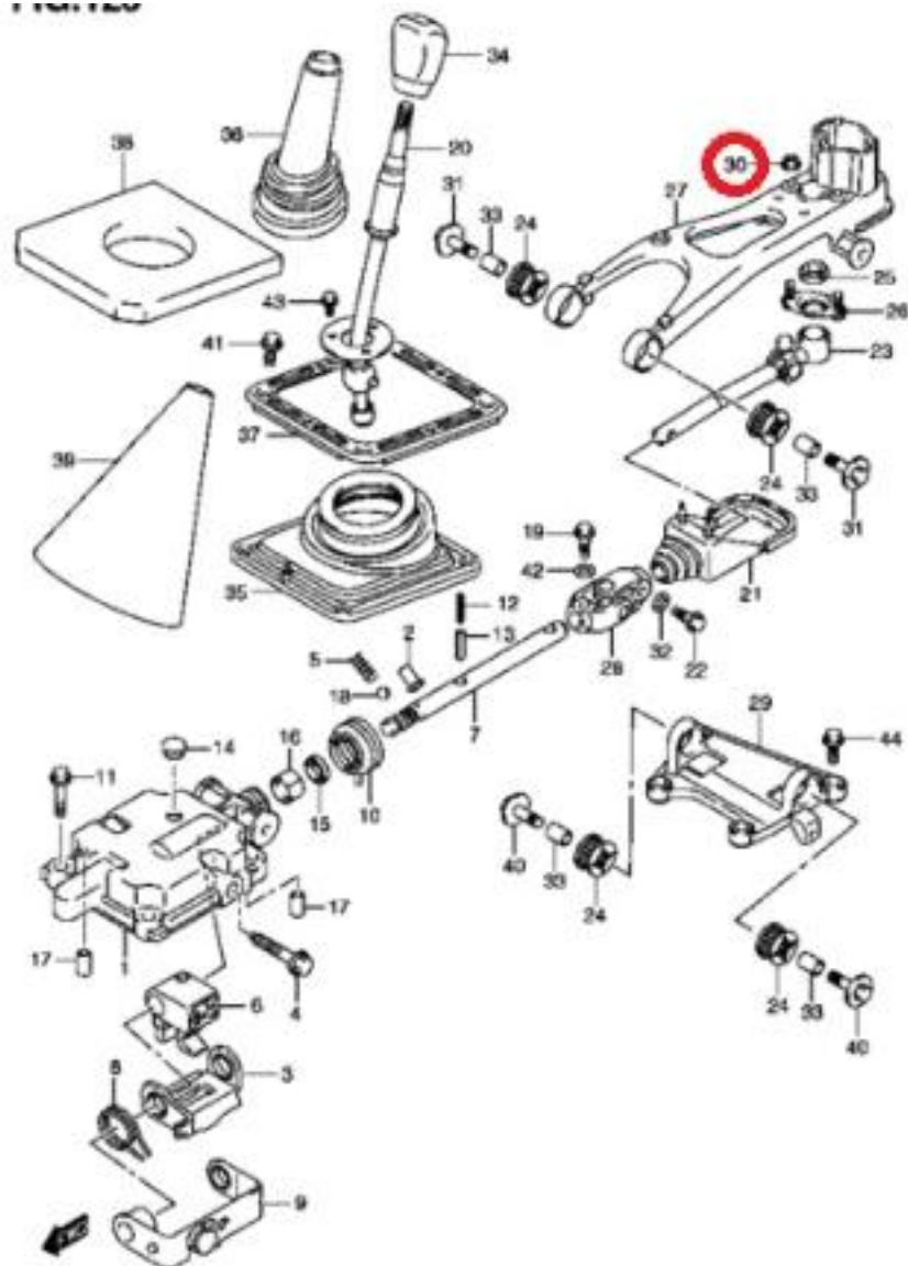
JB420W-4 E22_125 GEAR SHIFT CONTROL (1)
