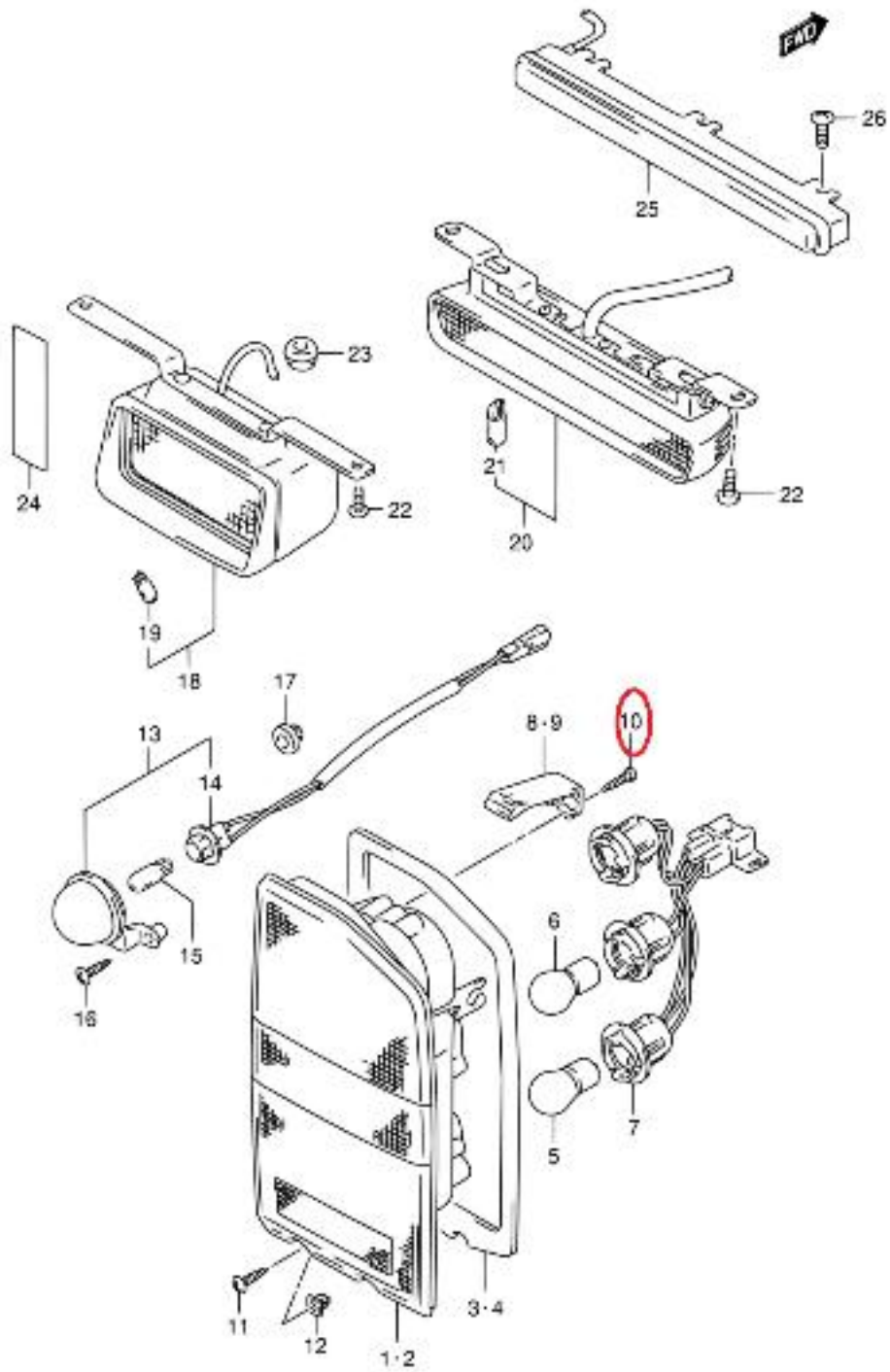
SE416-4 E01_118 REAR LAMP
