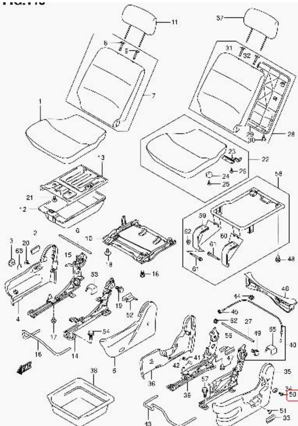
RC410 E35 1:0 FRONT SEAT(MT)
