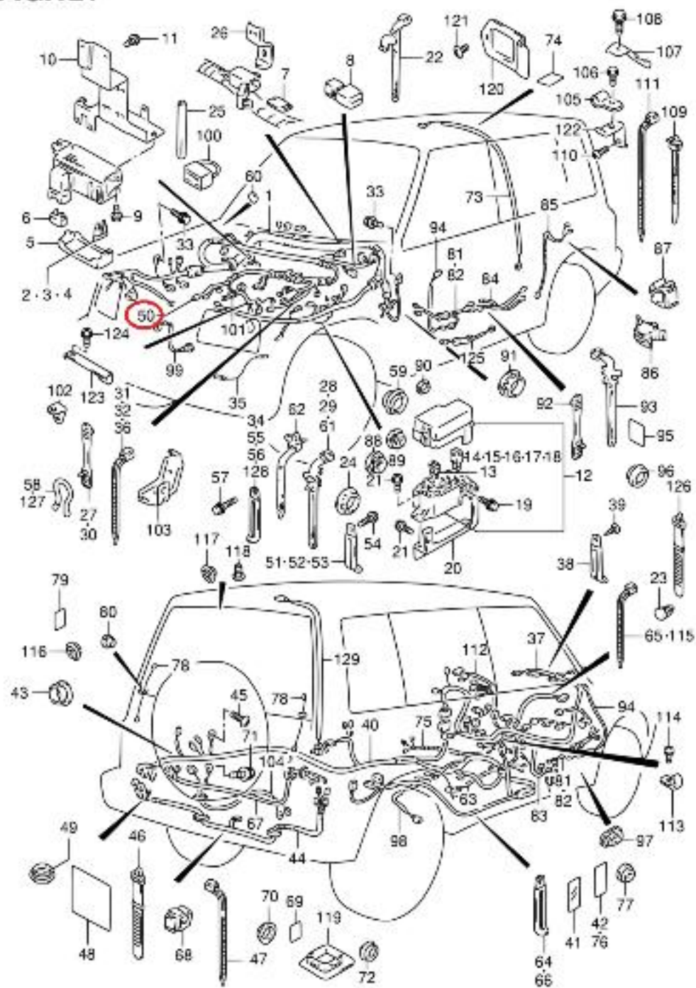
SE416-4 E01_121 WIRING HARNESS(RHD)
