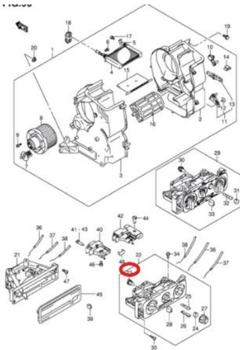
RA410 E10 E35_096 HEATER CONTROL (LHD)
