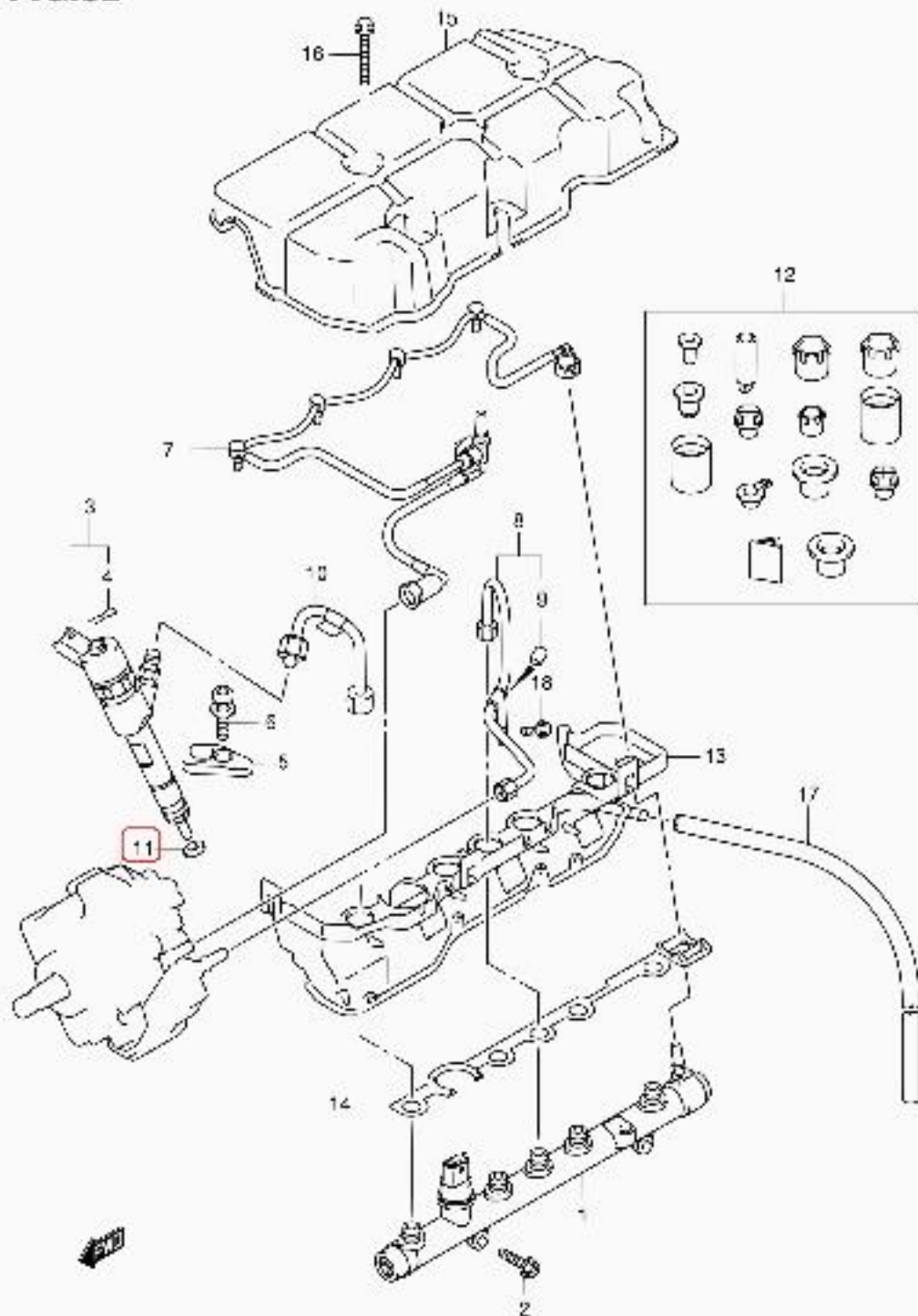
JB420W E22 032 DELIVERY PIPE (JB4'3)
