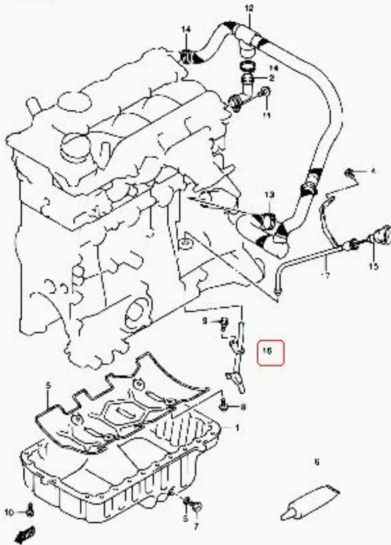
SQ420W-3 E22_510 OIL PAN (SQ420WD)
