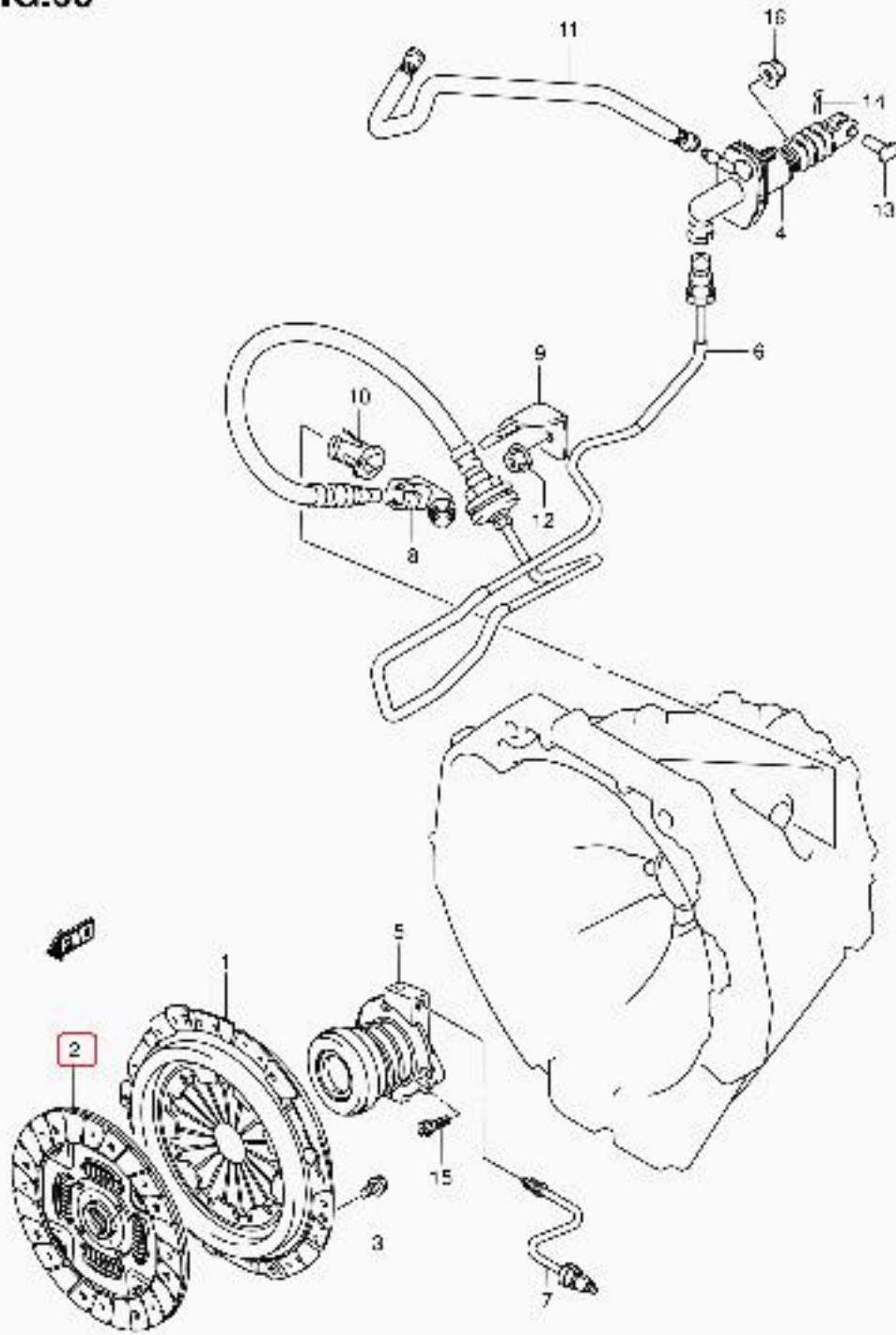
JB416X-4 E22 066 MT CLUTCH (1)
